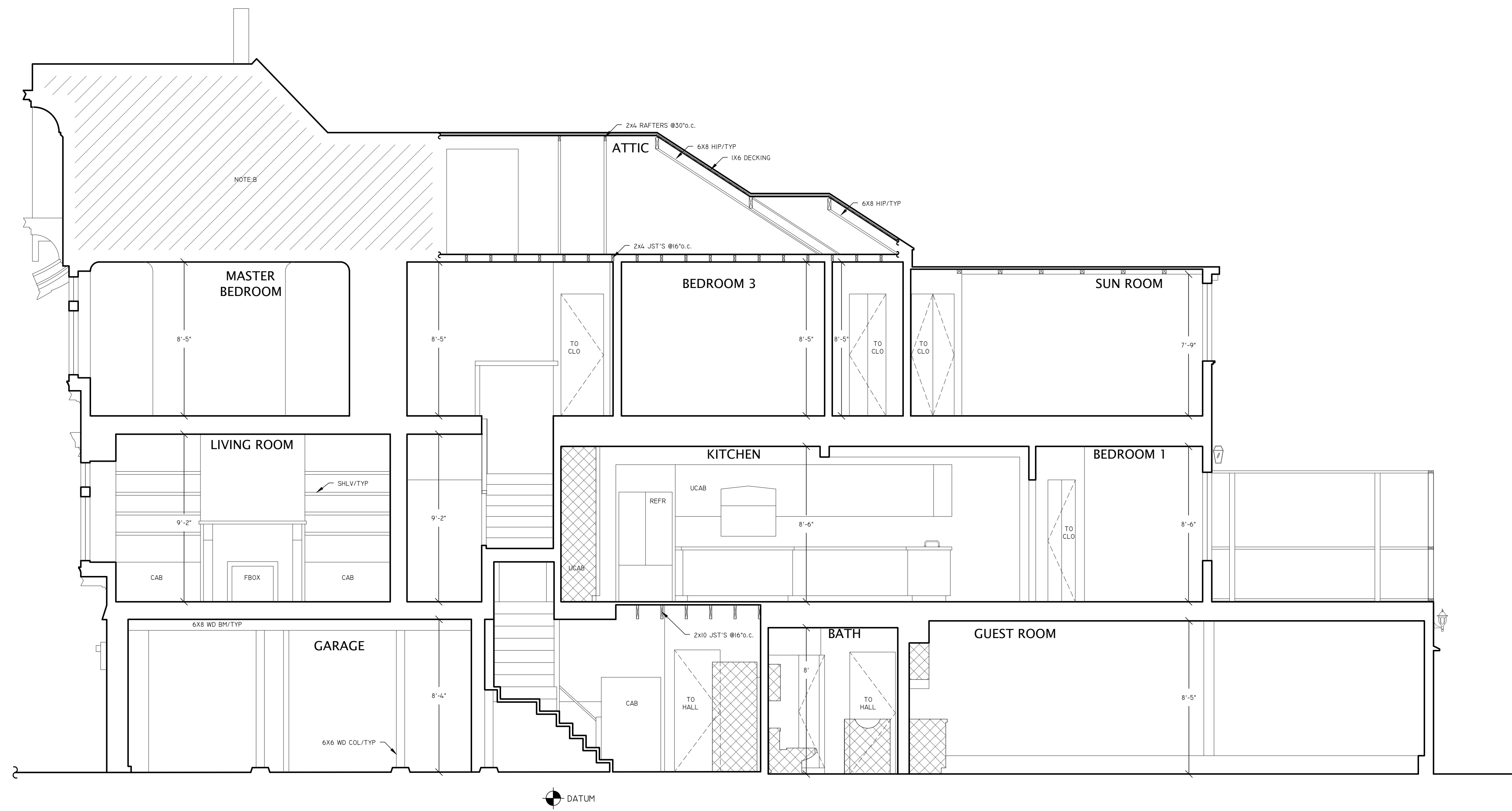
1 EXISTING LONGITUDINAL SECTION
